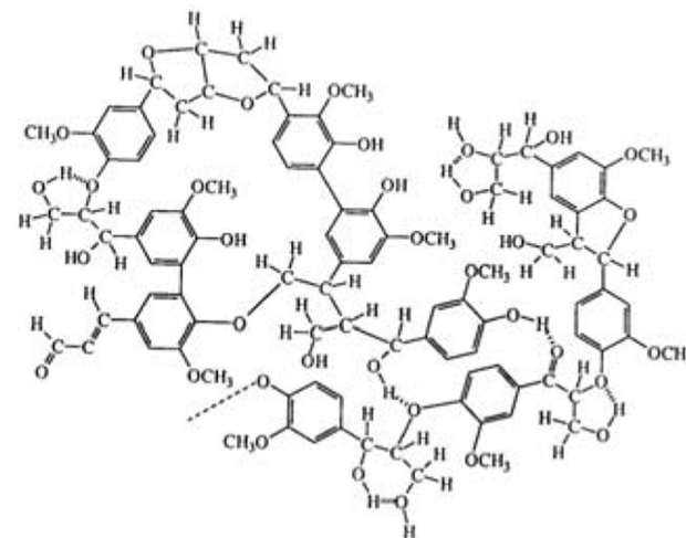
LIGNINA
